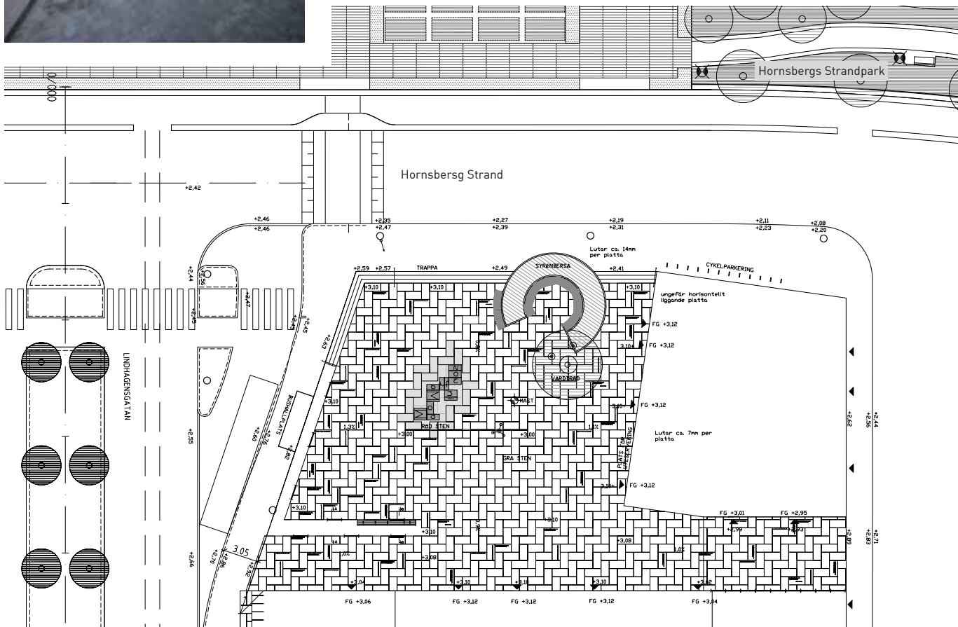
Moa Martinsons Torg, nordvästra Kungsholmen, Stockholm. Illustrationsplan Nyréns Arkitektkontor
