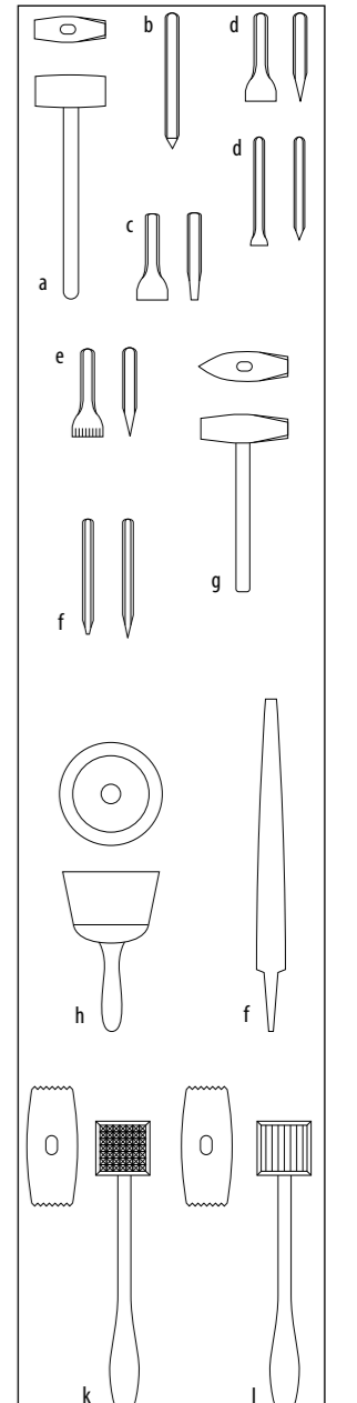
Fig 7.3 Lågerhuggning av kalksten med klubba och mejsel
