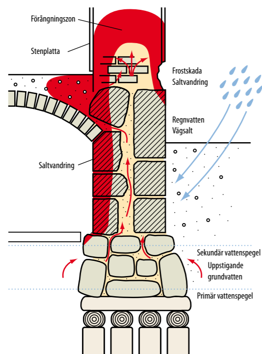
Fig 3.28 Saltvandring genom murverk.
