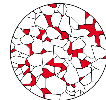
Fig 3.15 Kvarsbunden sandsten – kornen är kvarts eventuellt fältspat. Bindemedlet kvarts
