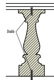
Fig 1.46 Balusterdocka fästad med dubb.
