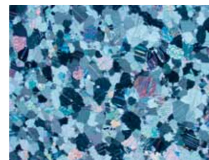
Fig 3.13 Marmor, tunnslip. Kalkspat eller dolomit med ensartad, "sockerkorning", kristallin textur. Verklig storlek: längd 5,5 mm.
