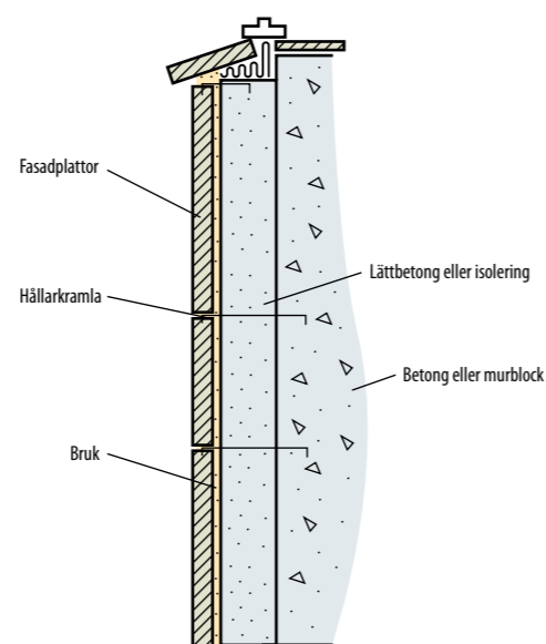
Fig 1.31 Principskiss av fasadplattor monterade i bruk och säkrade med hållarkramlor av tråd. Ibland användes även dubbar, ca \varnothing 10 mm, som bar plattorna i underkant.
