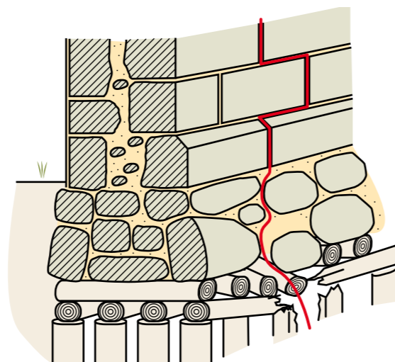
Fig 3.24 Exempel på rörelsebelastning och sättningar på grund av svårt rötskadade pålar.
