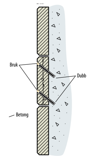
Fig 4.21 Principskiss för säkring av spjälkad platta med snedställda dubbr.
