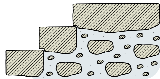
Fig 1.38 Den genom seklerna vanligast förekommande trappan har blocksteg lagda på grus och flissten.
